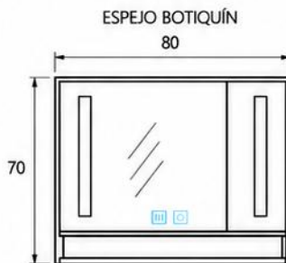
VISTA FRONTAL ESPEJO BOTIQUÍN
