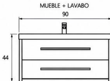
VISTA FRONTAL MUEBLE + LAVABO
