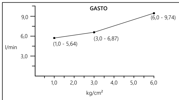
REGADERA MANUAL
