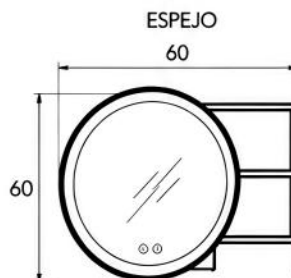
VISTA FRONTAL ESPEJO
