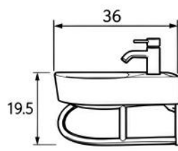
VISTA LATERAL MUEBLE + LAVABO
