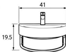
VISTA FRONTAL MUEBLE + LAVABO
