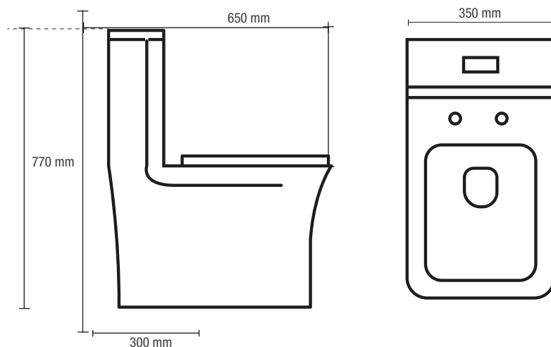
PLANO MECÁNICO
