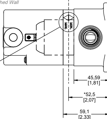
VISTA SUPERIOR (DETALLE DE INSTALACIÓN) TOP VIEW (INSTALLATION DETAIL)
