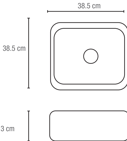
PLANO MECÁNICO
