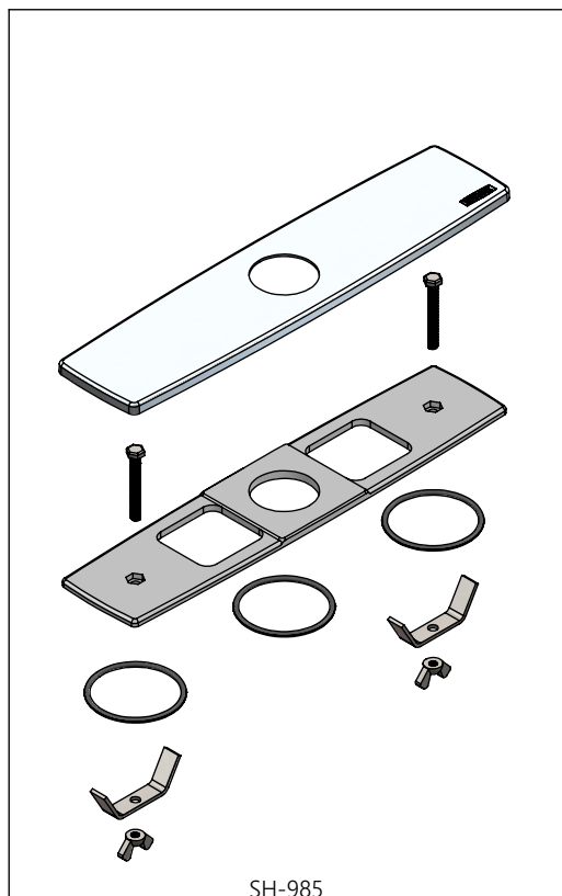
SH-985 Chapetón con Base y Sistema de Sujeción
