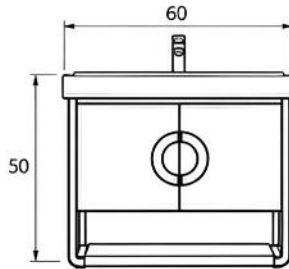
VISTA FRONTAL MUEBLE + LAVABO
