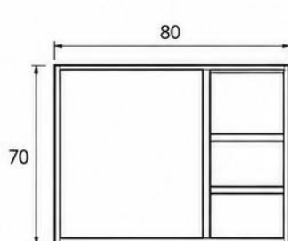
VISTA FRONTAL ESPEJO TIPO BOTIQUÍN
