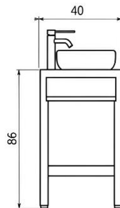
VISTA LATERAL
