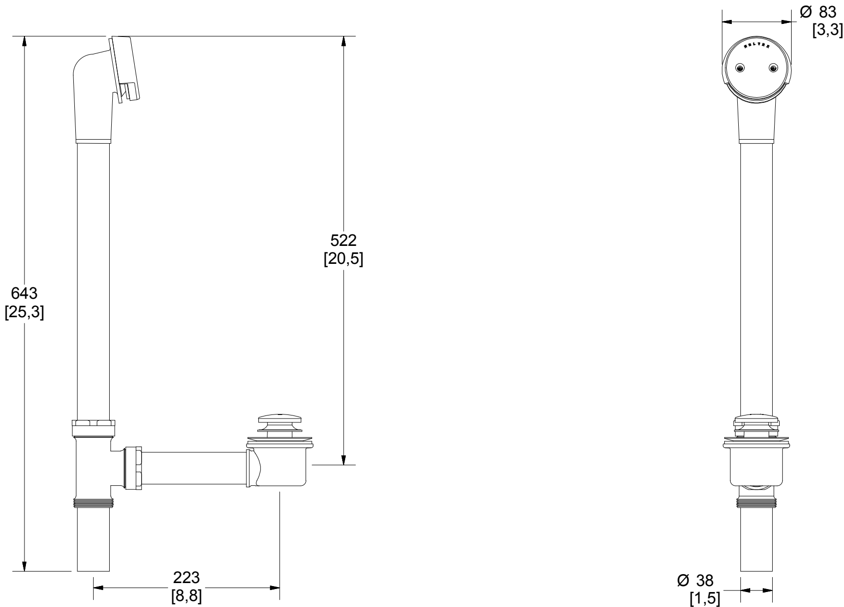
Medidas Referenciales / Estimated Dimensions, Acot. mm [pulg.] / Dim. mm [inch.]
