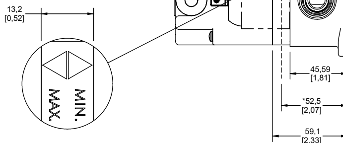
*DIMENSIÓN DE INSTALACIÓN RECOMENDADA * RECOMMENDED INSTALLATION DIMENSION
